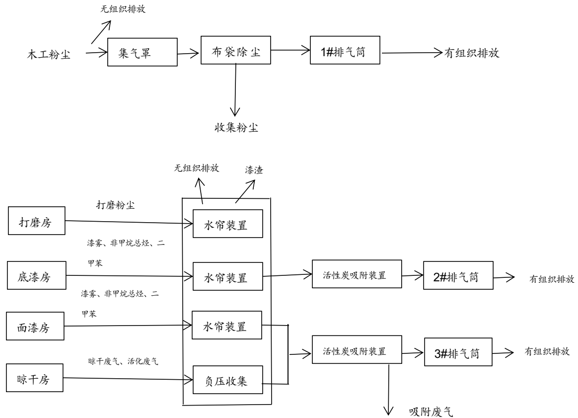
图 4-1 大气污染物收集处理走向图
