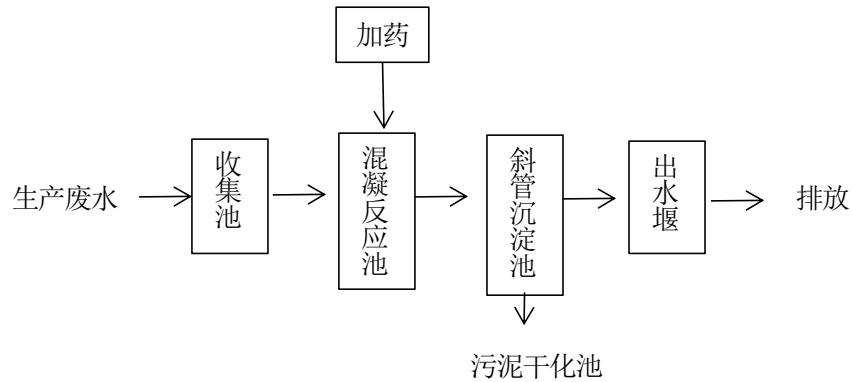
图 4-2 厂内污水处理站处理工艺
