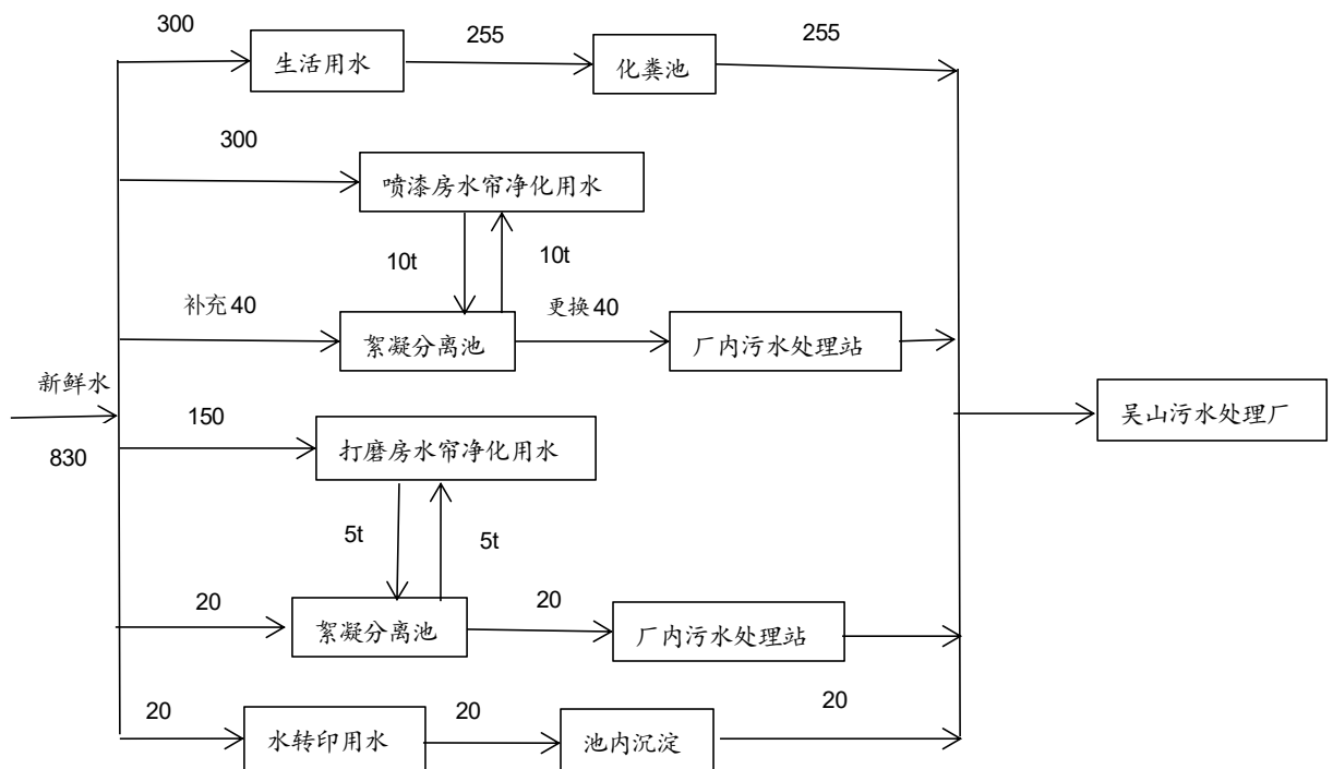
图 3-4 建设项目水量平衡图 (单位: t/a)
