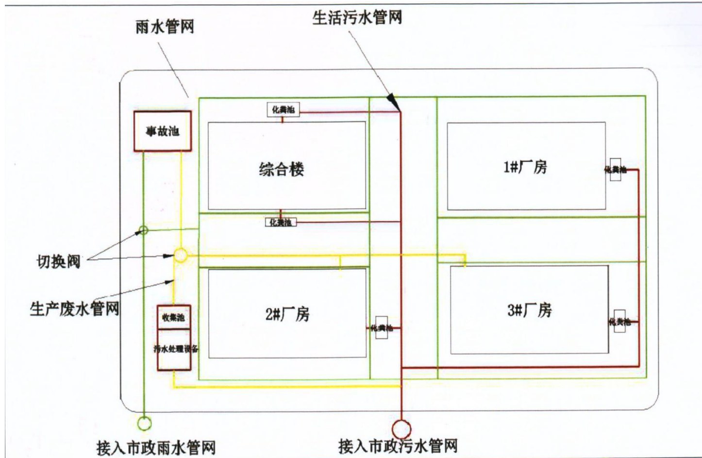
图 3-3 建设项目雨污管网
