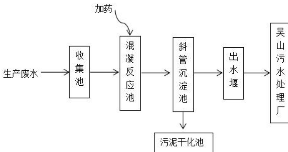
图 4-1 合资自建污水处理站工艺流程图
