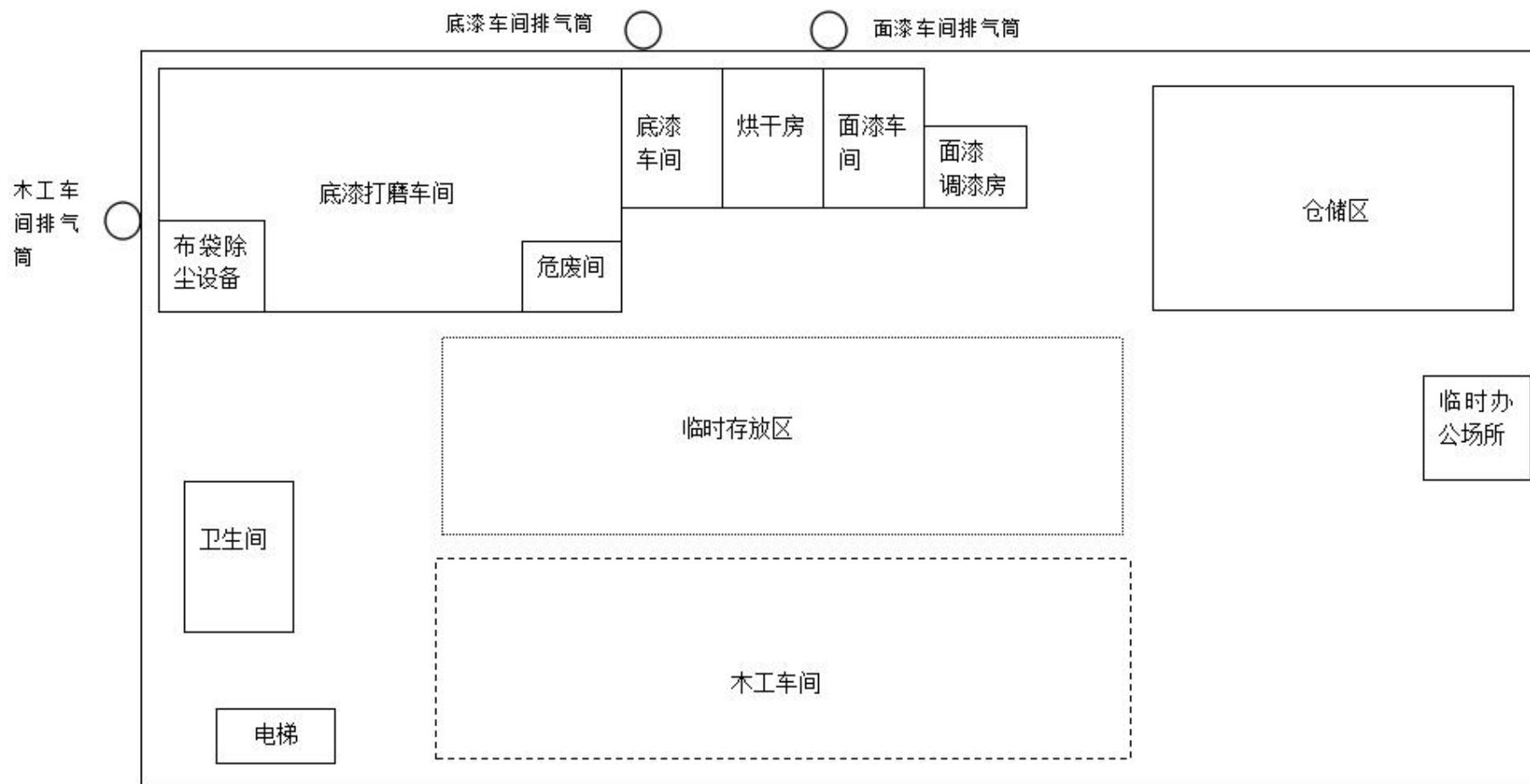
图 3-2 建设项目平面布置图
