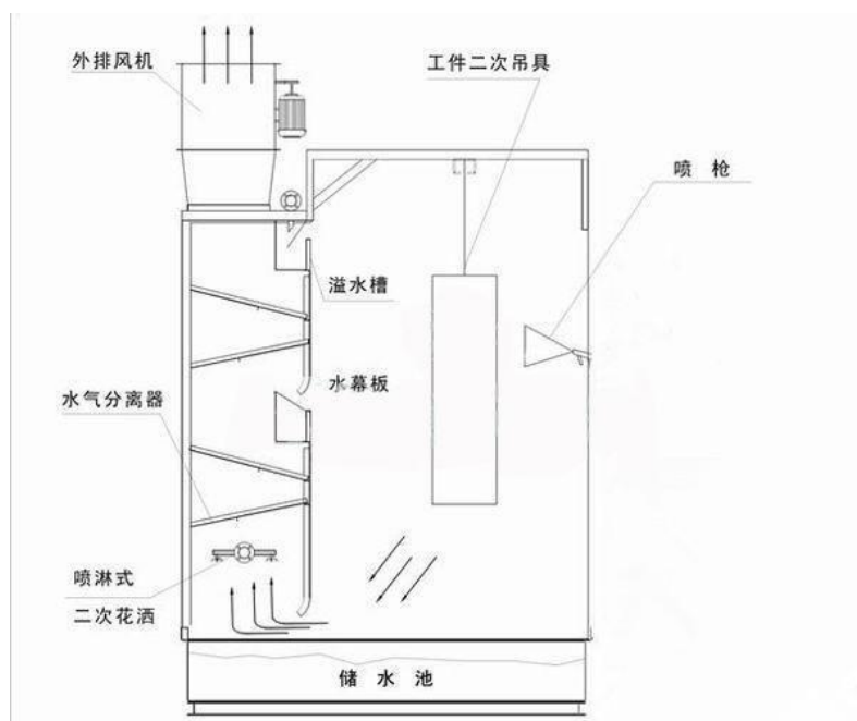
图 4-2 喷淋式水帘喷漆房工作原理图
