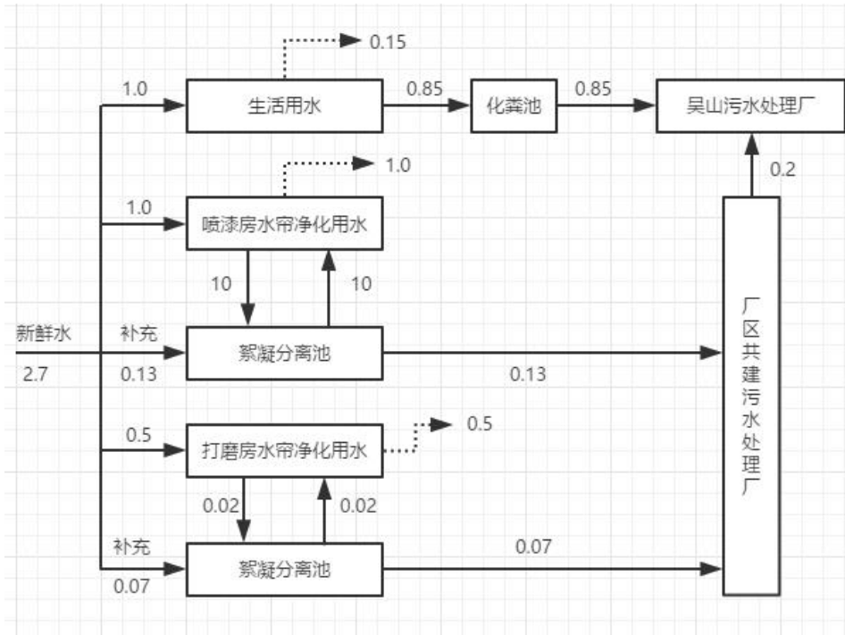
图 3-3 建设项目水平衡图 (t/d)
